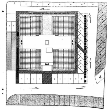
PLANIMETRIA AREA ESTERNA - scala 1:4m
